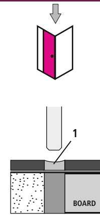
3 Zementfuge / Joint en ciment / Cement joint / Cementvoeg / Fuga di cemento / Junta de cemento / Spoina cementowa / Cementová spára / Cementová medzera / Цементный шов / 水泥缝 / Cementfog / Cementfuge / Cement fuga
