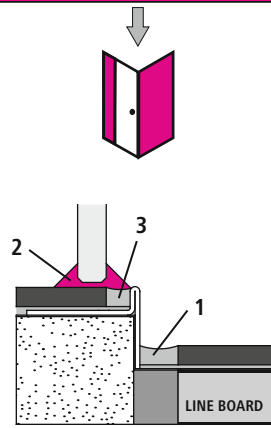
2 Versiegelung / Scellement / Sealing / Siliconen-kitnaad / Sigillatura / Sellado / Uszczelnienie zewnętrzne / Uzavírací náter / Tesniaca hmota / Герметик / 密封胶 / Försigling / Forsegling / Elzárás
